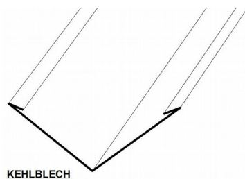
Masskantenteile max. Kantlänge 2,5 Meter
