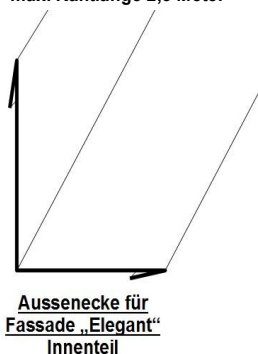
Masskantteile max. Kantlänge 2,5 Meter
