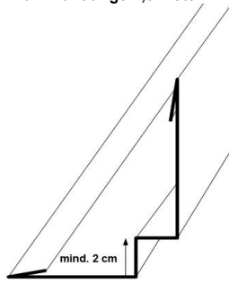
INNENECKE für Fassade „Elegant“
