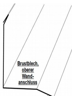
Masskantenteile max. Kantlänge 2,5 Meter
