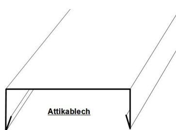
Masskantenteile max. Kantlänge 2,5 Meter
