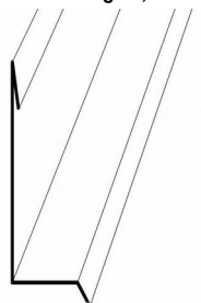
Wandanschluss – Trapezblech in Verbindung mit Kittleiste
