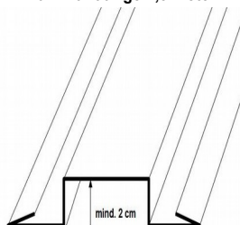
HUTPROFIL Stossverbinder für Fassade „Elegant“
