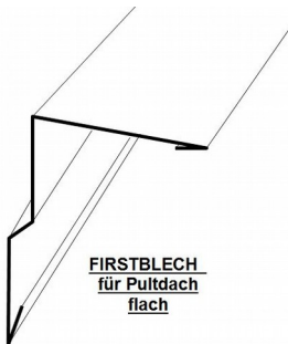
Masskantenteile max. Kantlänge 2,5 Meter
